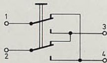
Schaltbild des Polwendeschalters
